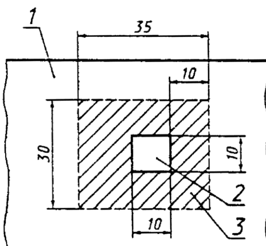
Рисунок Б.2 - Схема проведения надреза для сдвига образца покрытия
